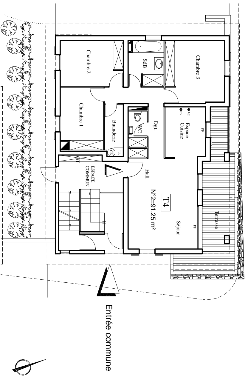
Plan du 1er Etage
