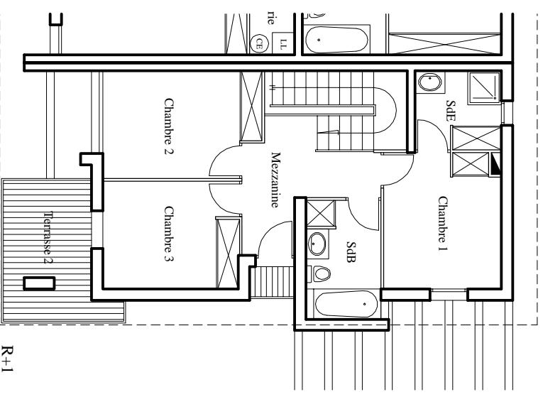
Plan du Niveau 1
